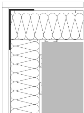
Metselwerk muur
